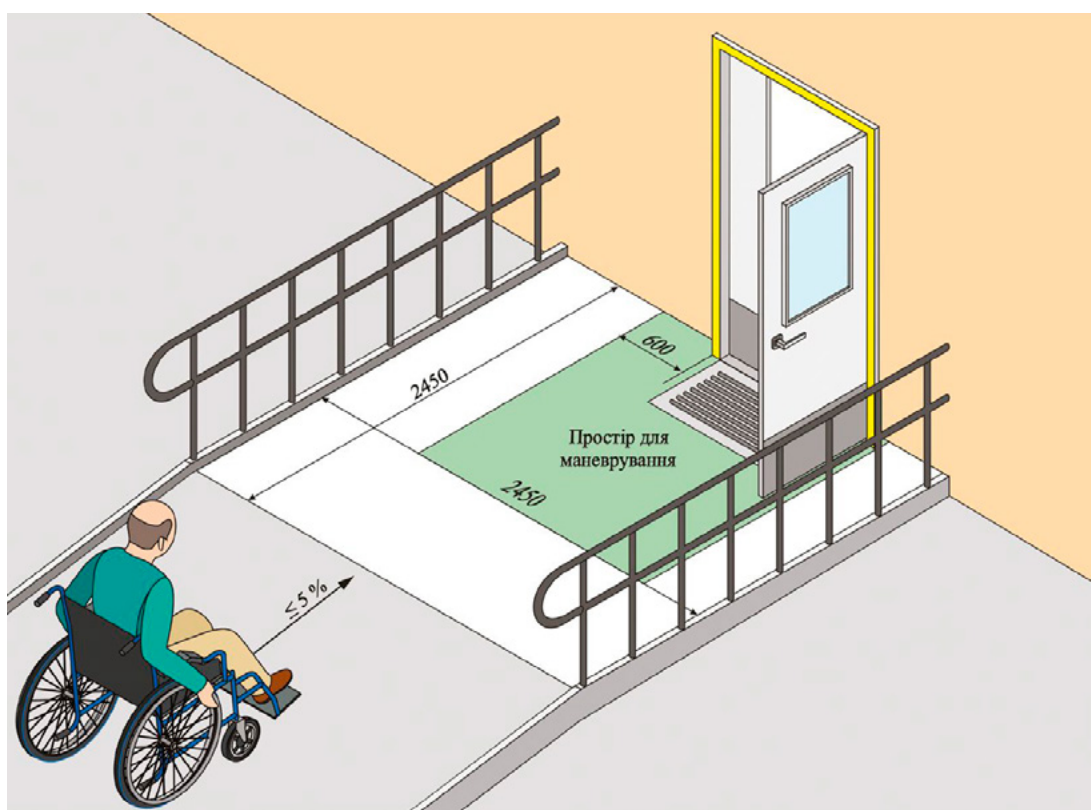
Рис. 5. Вхідна зона без ґанку
