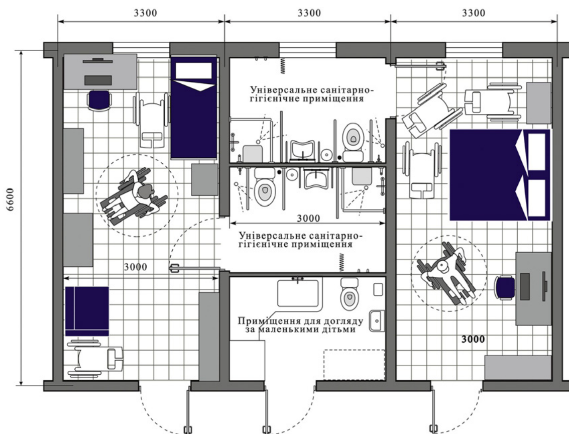
Рис. 17. Схема житлових приміщень з універсальним санітарно-гігієнічним приміщенням на кожну кімнату
