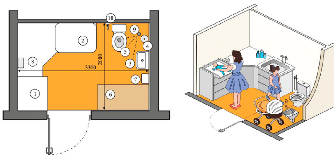
Рис. 20. Схема обладнання приміщення для догляду за маленькими дітьми
