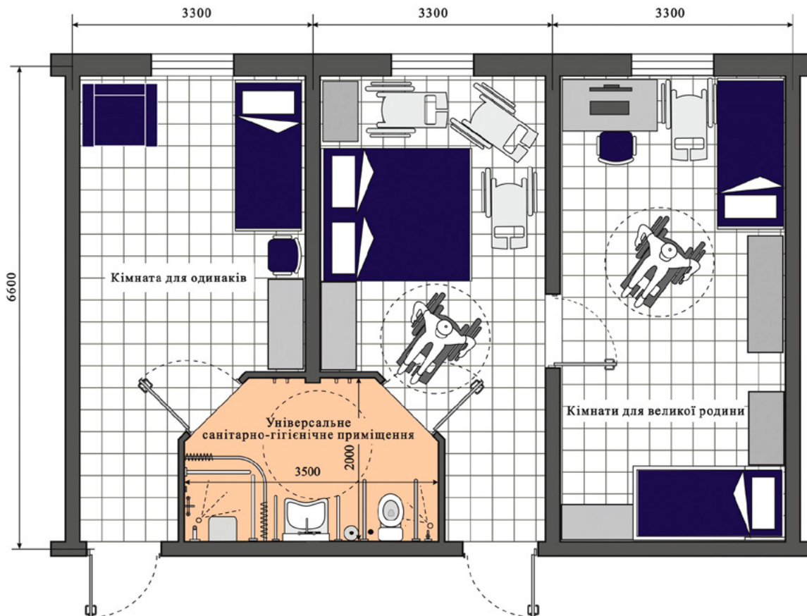
Рис. 15. Схема житлових приміщень з універсальним санітарно-гігієнічним приміщенням на суміжні кімнати
